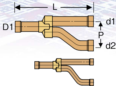
3系列(黄铜Y型分歧管)
